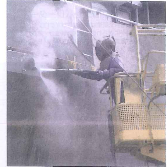
▼混気ジェット 水ブラスト状況
